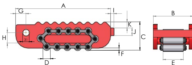
Эскизы моделей RSN60 и RSN80
