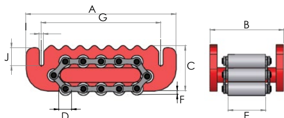
Эскизы моделей RSN10, RSN15 и RSN30
